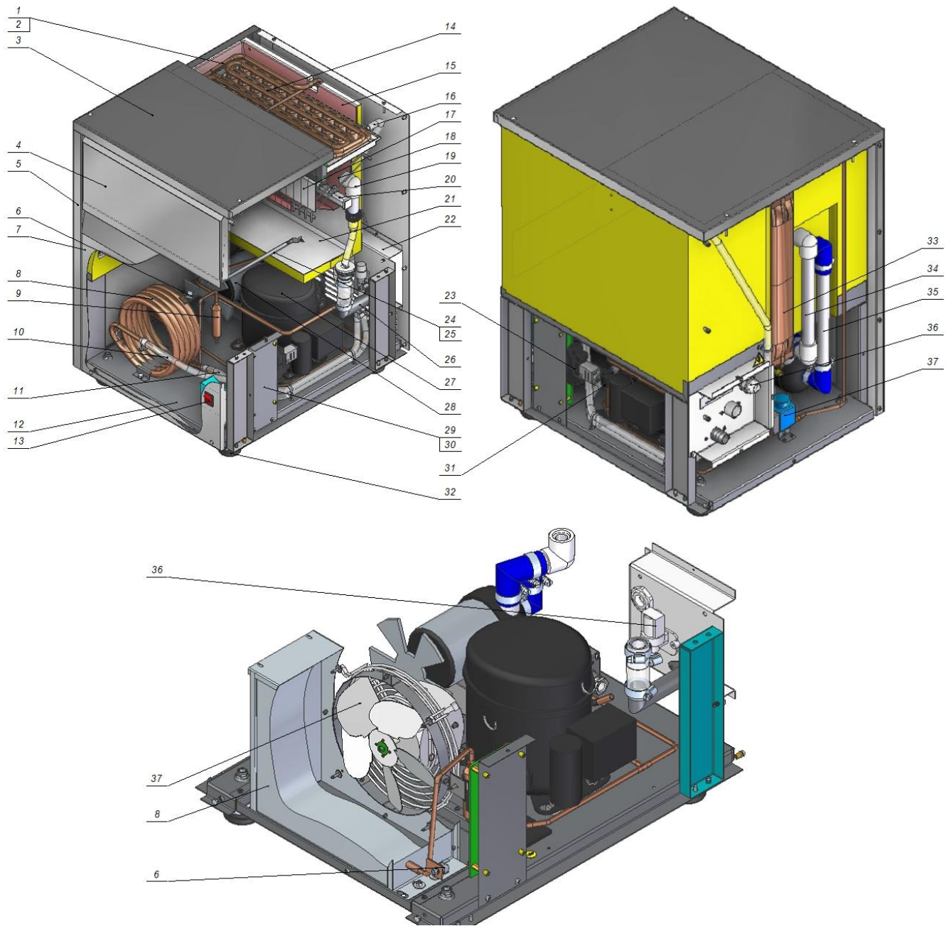
Рис. 1 Устройство льдогенераторов
