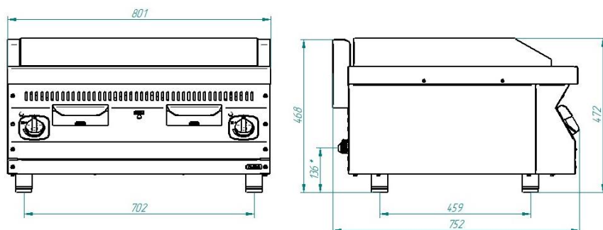
Рис. 3 - Общий вид ЭГЛ-80/2Н-00, где * - подвод электропитания
