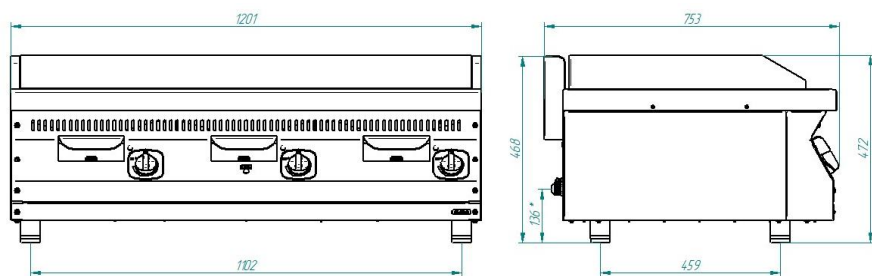
Рис. 5- Общий вид ЭГЛ-120/3Н-00, где * - подвод электропитания
