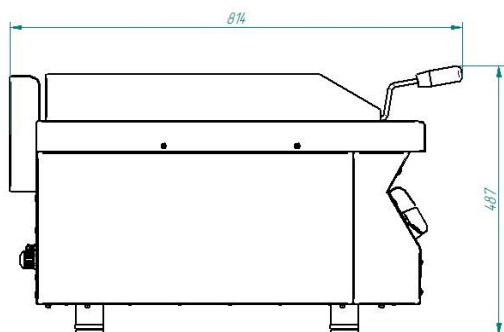
Рис. 4 - Общий вид ЭГЛ-80/2Н-01, остальное см.рис.3
