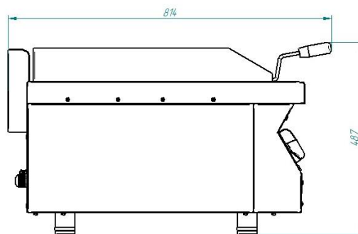
Рис. 2 - Общий вид ЭГЛ-40/1Н-01, остальное см.рис.1
