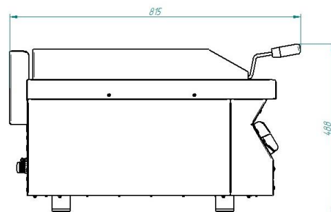
Рис. 2 - Общий вид ЭГЛ-120/3Н-01, остальное см.рис.1
