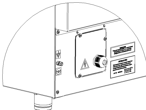
Рис. 4 - Место подключения ЭГЛ-40/1Н-00, ЭГЛ-40/1Н-01, ЭГЛ-80/2Н-00, ЭГЛ-80/2Н-01, ЭГЛ-120/3Н-00, ЭГЛ-120/3Н-01
