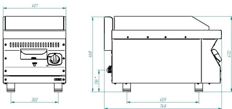
Рис. 1 - Общий вид ЭГЛ-40/1Н-00, где * - подвод электропитания
