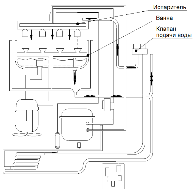
Рис. 2 Отличия льдогенераторов ЛГ-24/06К-02П, ЛГ-24/06К-04П
