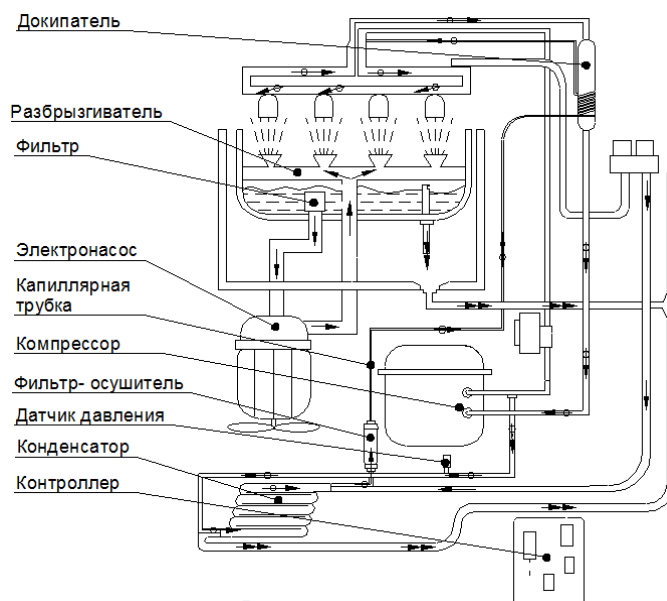
Рис. 2 Отличия льдогенераторов ЛГ-24/06К-02П, ЛГ-24/06К-04П
