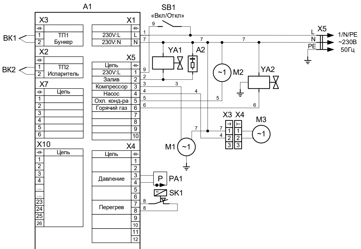
Схема электрическая соединений ЛГ-24/06К-01П, ЛГ-24/06К-03П
