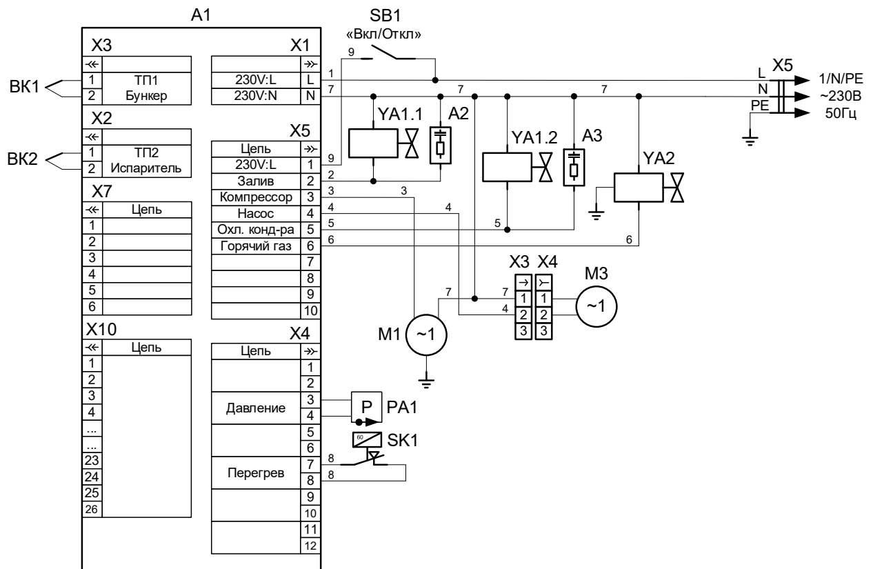
Схема электрическая соединений ЛГ-24/06К-01П, ЛГ-24/06К-03П
