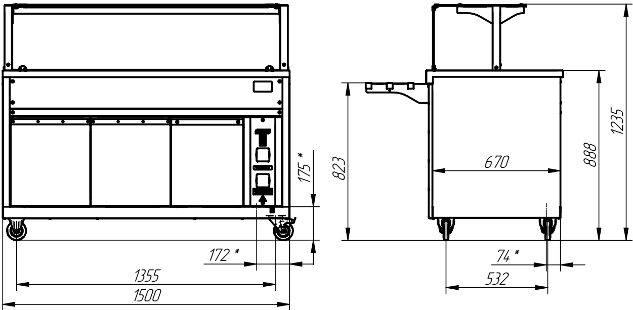
Вариант с поворотными колесами
