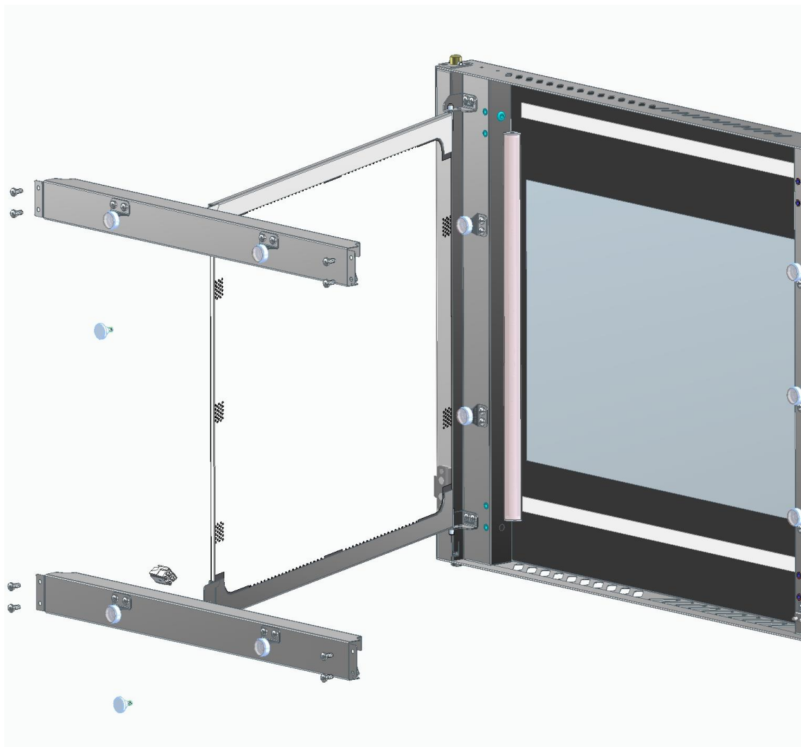
Рис. 23 Замена ламп освещения
