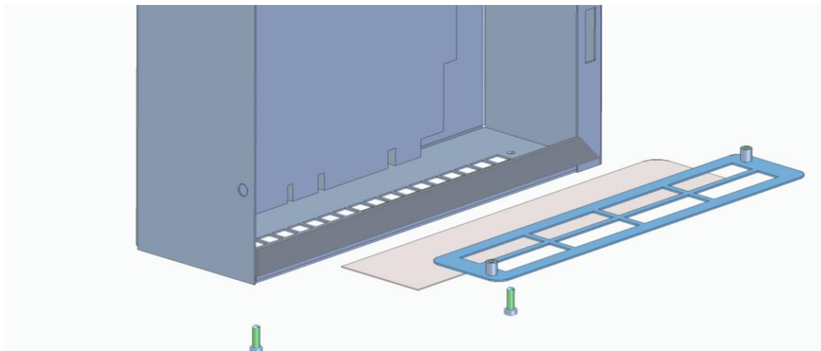
Рис.24 Замена воздушного фильтра
