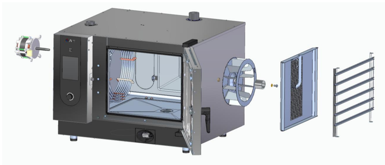
Рис. 17 Схема замены манжет
