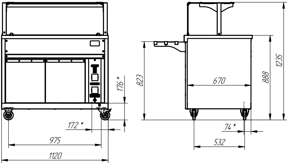
Вариант с поворотными колесами
