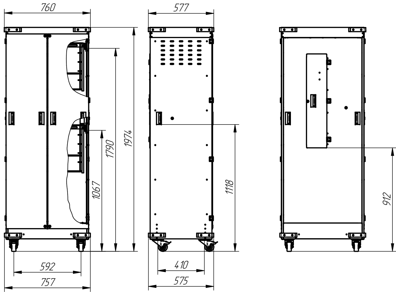
Тележка загрузочная ТЗ-10-6-4 с кассетами 5 + 5 уровней
