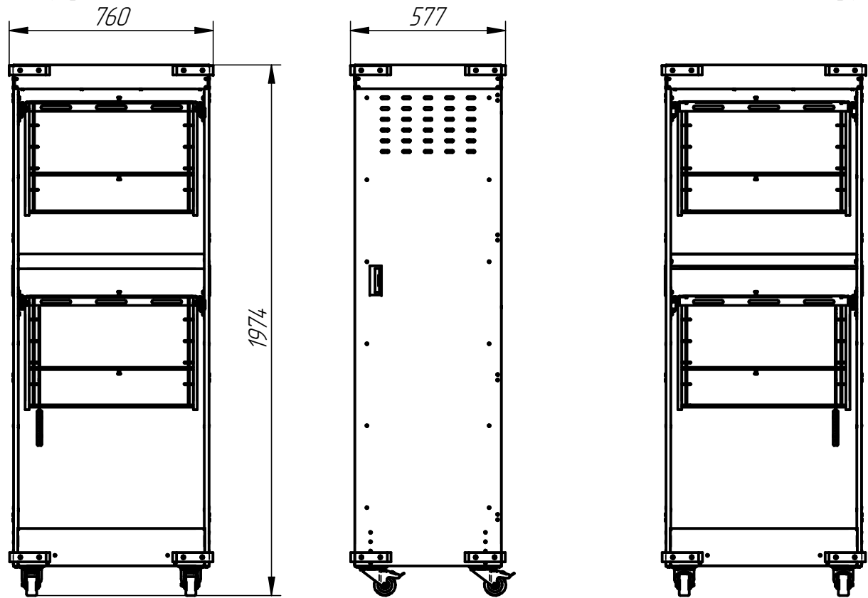
Тележка загрузочная ТЗ-10-6-4 (открытая) с кассетами 5 + 5 уровней
