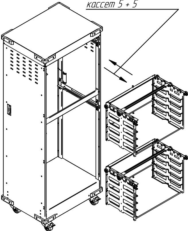
Загрузка и выгрузка кассет 5 + 5
