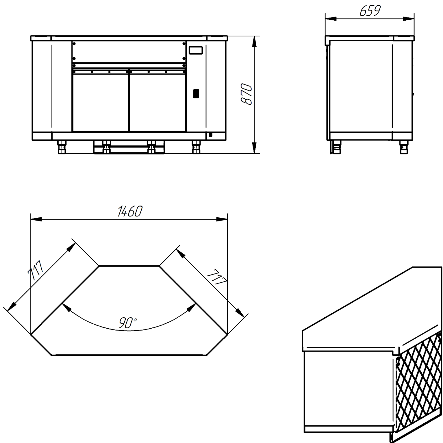
Рис.5 Общий вид.
